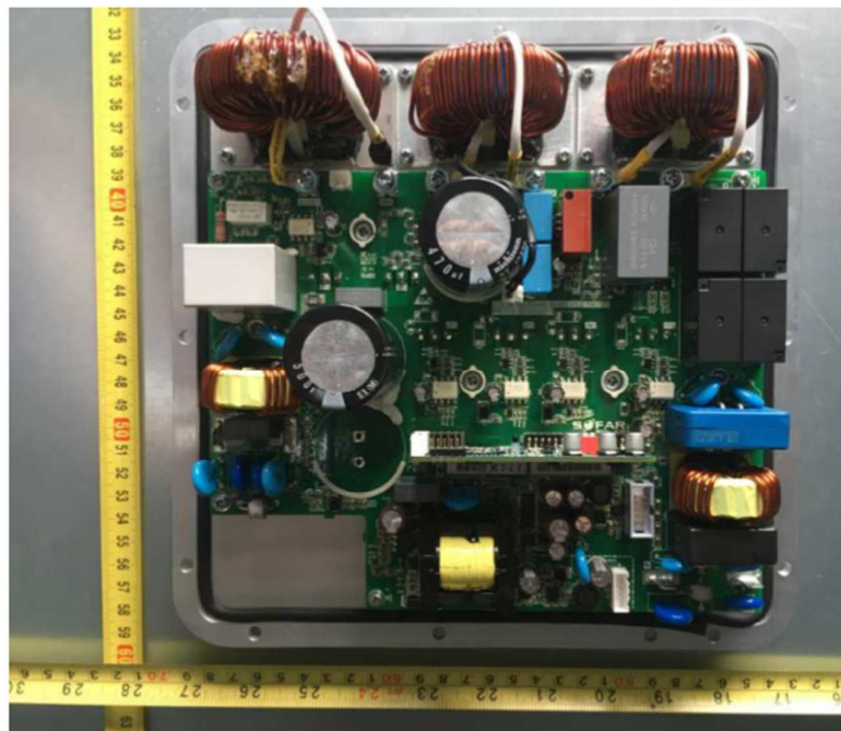
Figura 3, Visão interna Figure 3, Internal view
